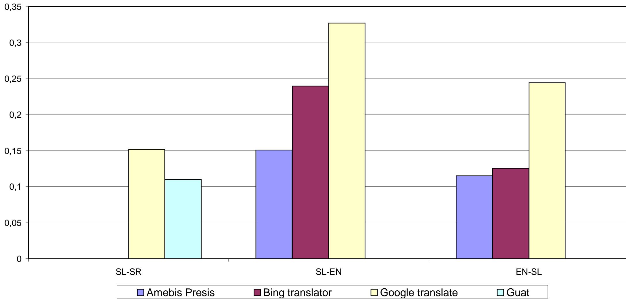
Vrednosti metrike BLEU
